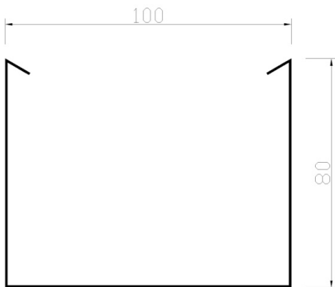
Profilsnitt genom skenan
